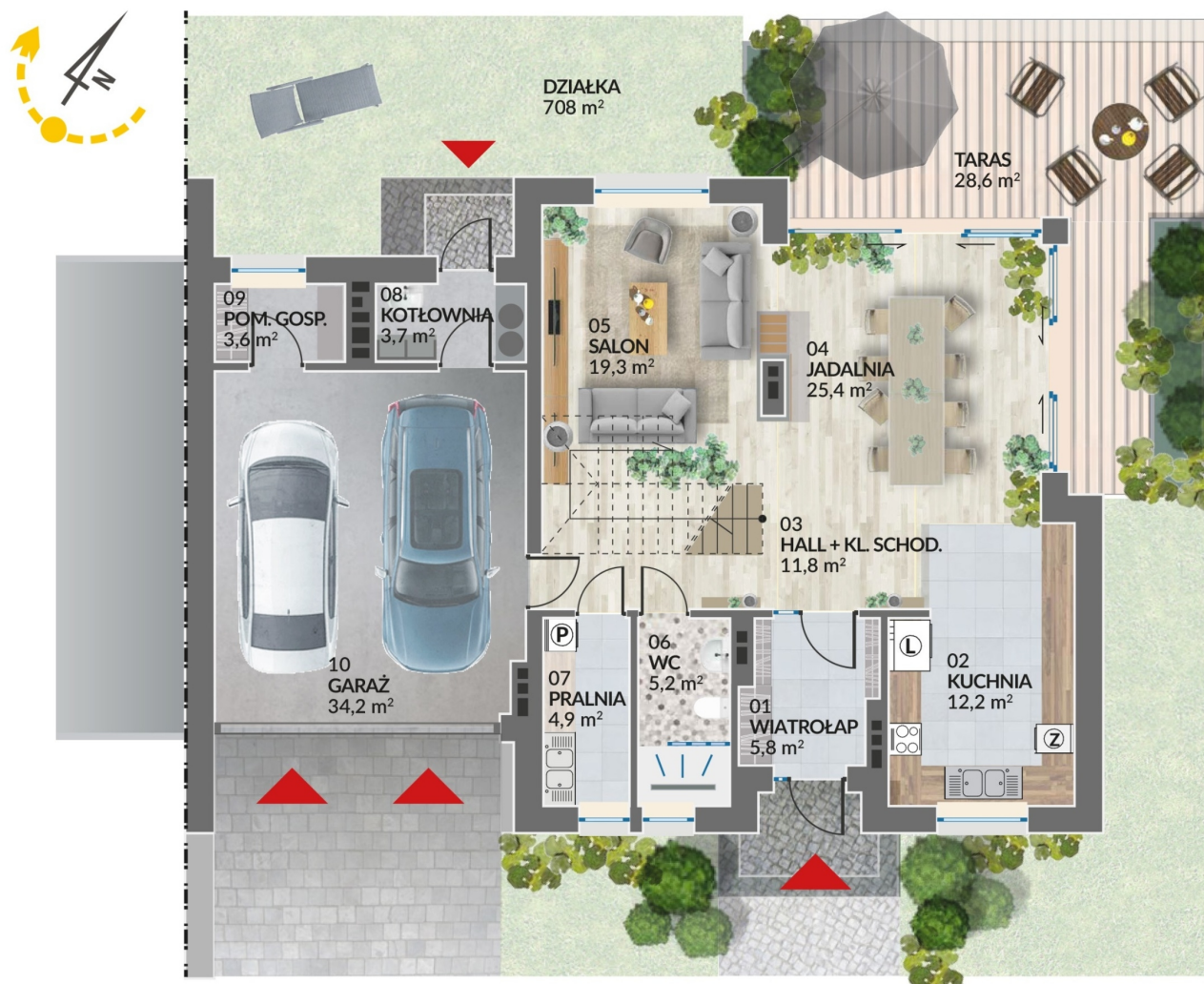
Rzut parteru
