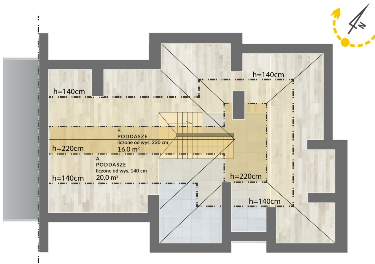
Rzut poddasza
