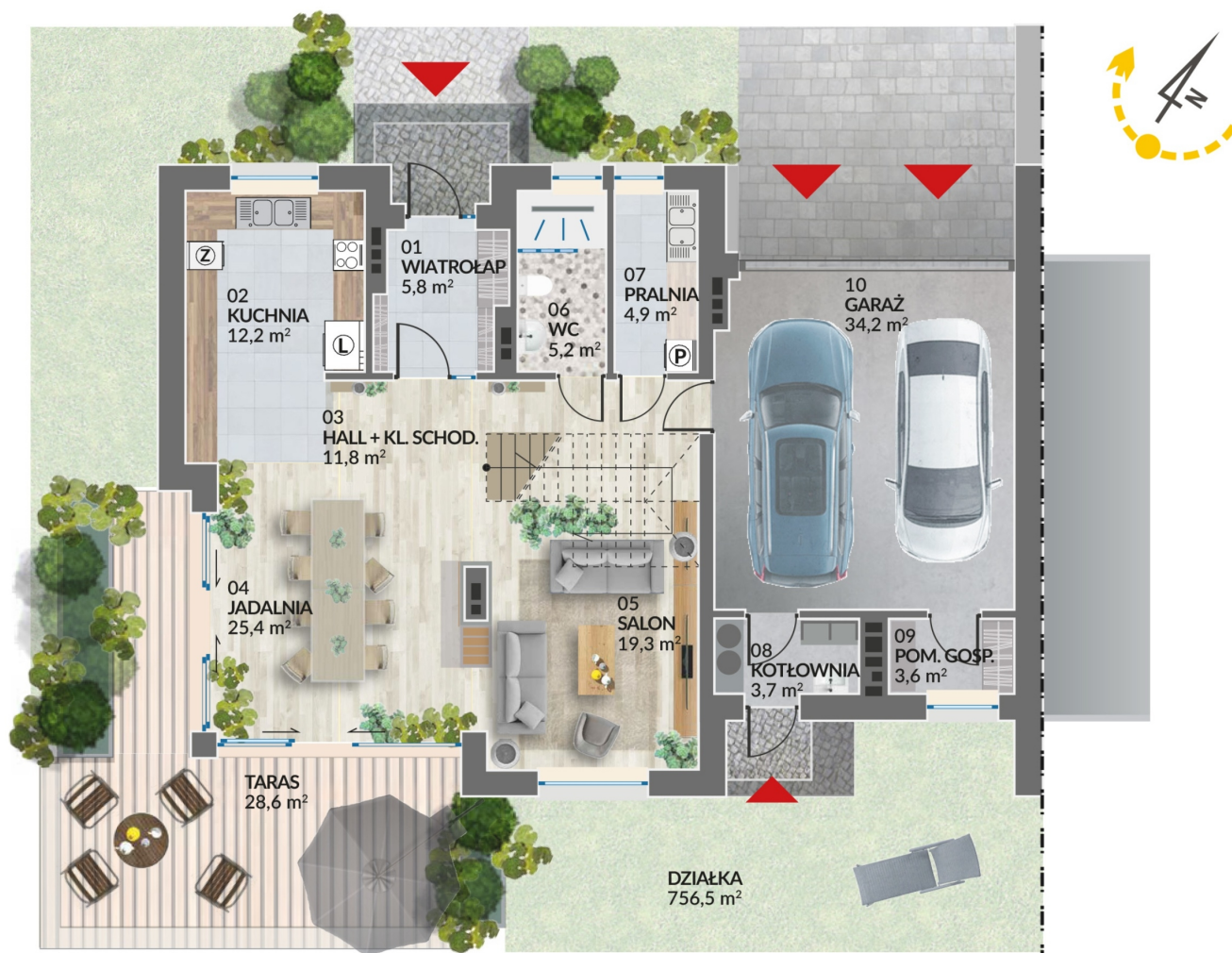
Rzut parteru
